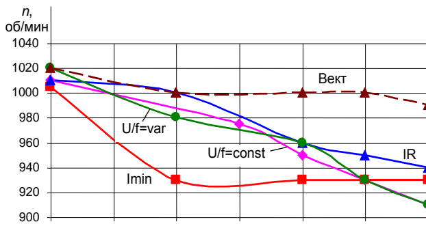
Рис. 2 Механические характеристики ( f=50 Гц)
