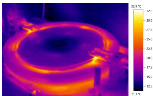
Рис.3. Теплограма зразка №1.
